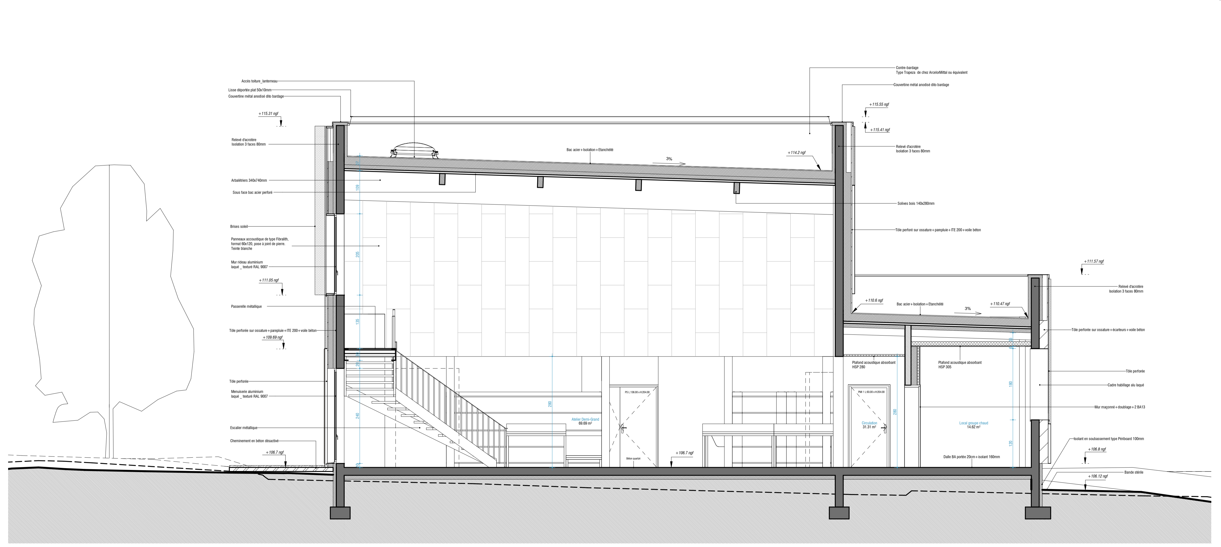
COUPE TRANSVERSALE EE'
