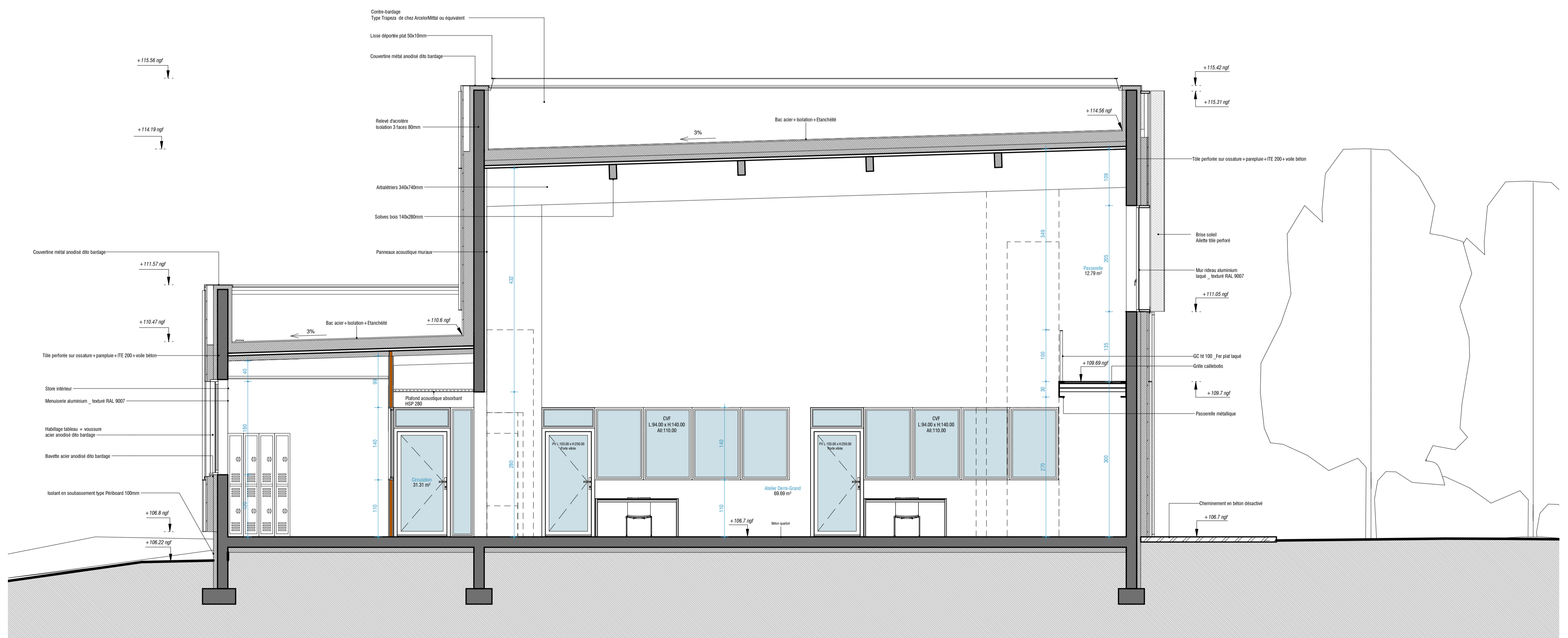
COUPE TRANSVERSALE DD'
