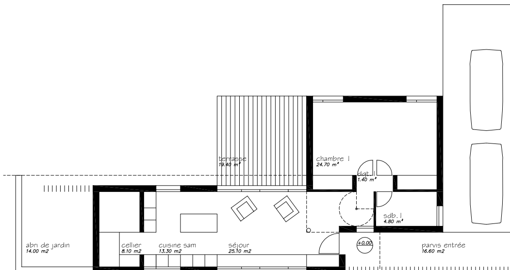
plan RDC
