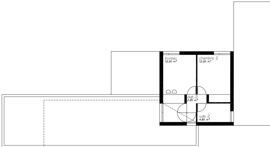
plan ETAGE 1
