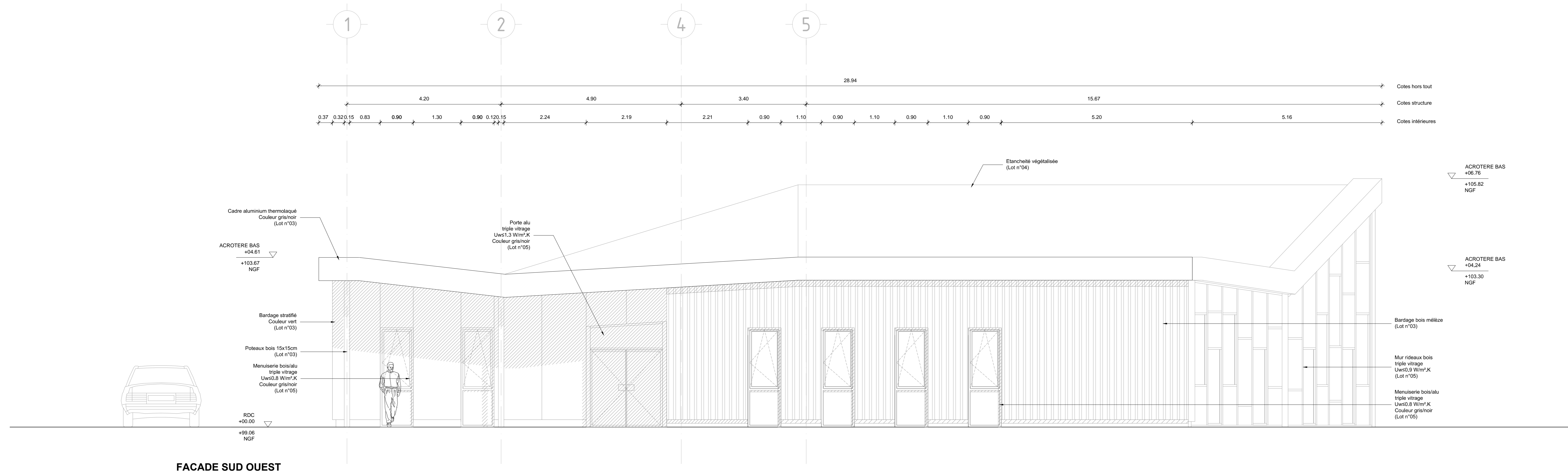
FACADE SUD OUEST
